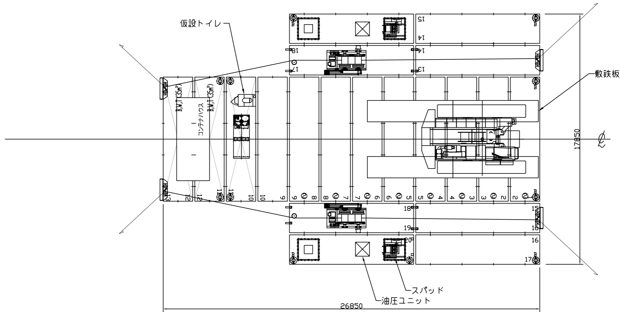
20基接続 ウインチ&スパッド艀装図
